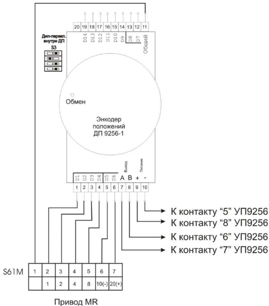
Рисунок А.9 – Подключение ДП 9256-1 к приводу MR для работы с VCD-сигналом или с произвольными комбинациями контактов (тип датчика «ДП9256 пользовательский» - код датчика 7);
