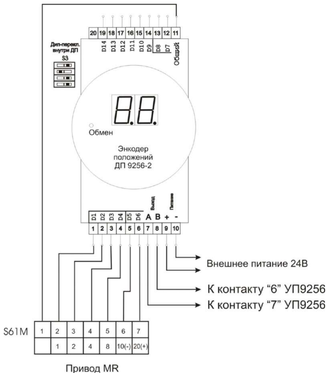
Рисунок А.10 – Подключение ДП 9256-2 к приводу MR для работы с VCD-сигналом или с произвольными комбинациями контактов (тип датчика «ДП9256 пользовательский» - код датчика 7);
