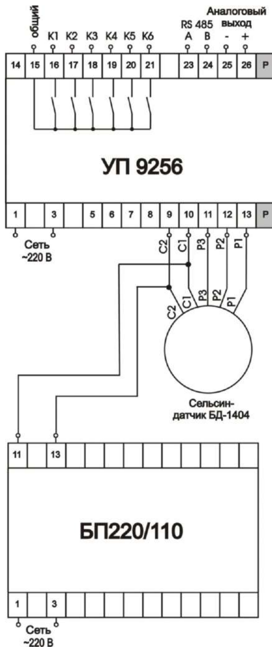
Рисунок А.8 – Схема электрическая подключения УП (питание ~220 В ±10 %) к сельсин-датчику (питание ~110 В) совместно с БП220/110.
